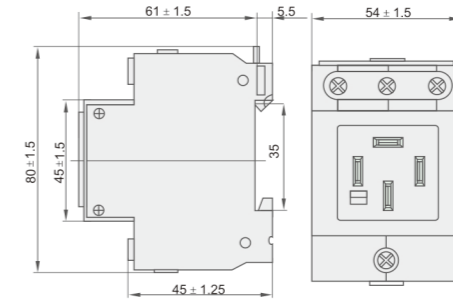
3P+接地 16A
