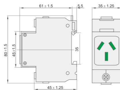
2P+ 接地 10A、16A
