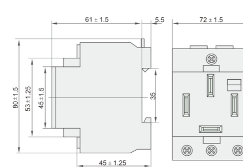
3P+接地 25A
